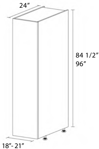
1 DOOR • 4 SHELVES R: RIGHT L: LEFT
